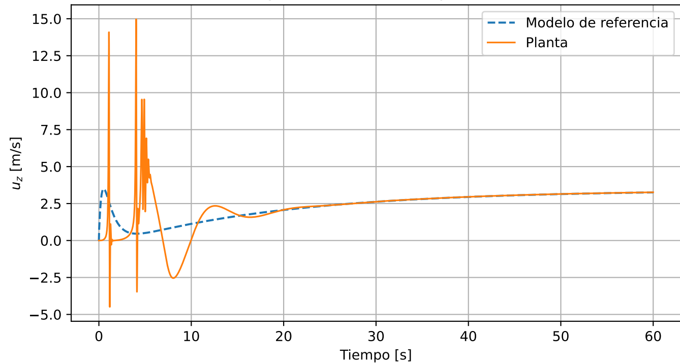
Seguimiento MRAC con paso: uz
